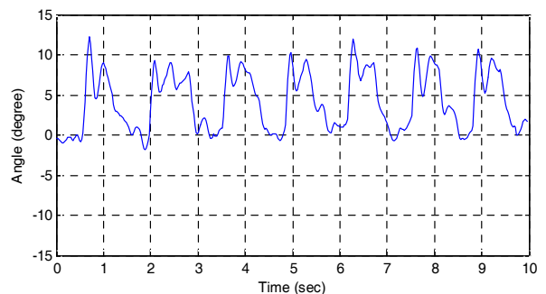
그림 11. PD 제어기 외란 실험. Fig. 11. PD control results to disturbance.
