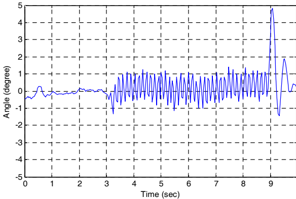
그림 12. Ohnishi의 DOB 실험 자세 데이터. Fig. 12. Ohnishi's DOB scheme.
