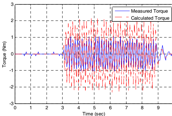
그림 13. 그림 12의 토크. Fig. 13. Torque of Fig. 12.
