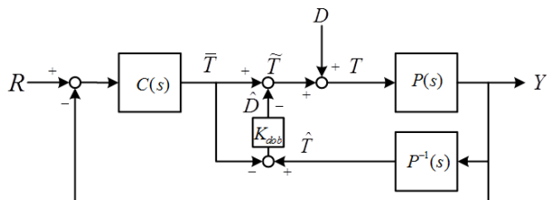
그림 3. 변형된 DOB 구조. Fig. 3. Modified DOB structure.
